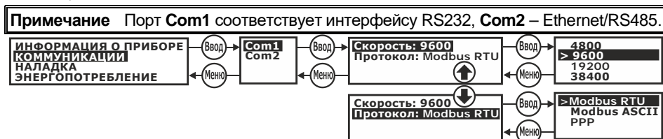
Рис. 3.13 – Настройка Com-портов
